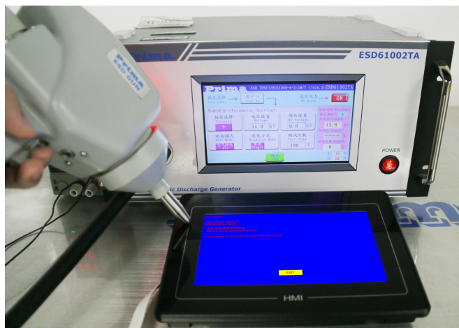
图 7-2 ESD 测试图
