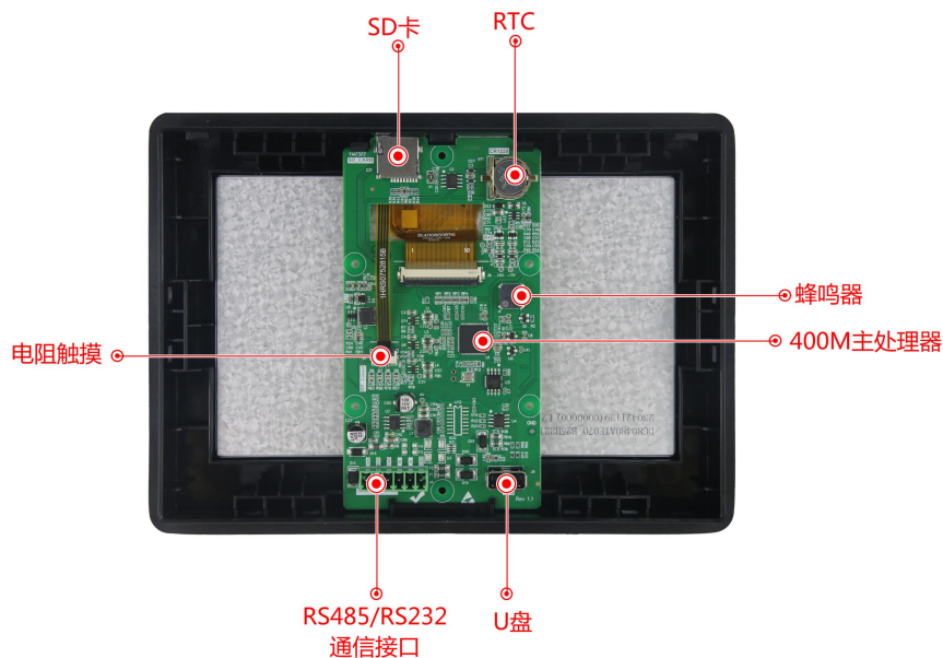
图 1-2 硬件配置图
