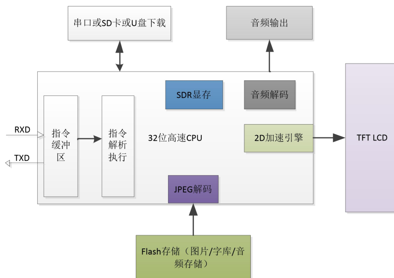
图 11-1 HMI 硬件结构参考图
