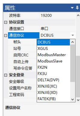
图 3-1 PLC 协议
